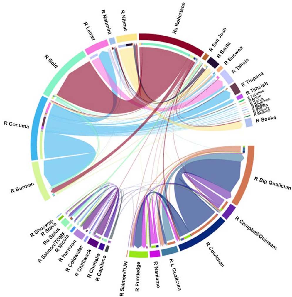
Figure 2. Diagramme à cordes du total des récupérations élargies de poissons égarés observées dans le sud de la Colombie-Britannique (à l'aide des données thermiques et des micromarqueurs magnétisés codés) entre 1998 et 2021 pour les réseaux hydrographiques récepteurs. La bande la plus externe présente les rivières donneuses dans le sud de la Colombie-Britannique; la couleur de la bande intérieure correspond à celle du réseau hydrographique récepteur, la direction et l'épaisseur des flèches indiquent le sens et l'ampleur de l'égarement à partir des réseaux hydrographiques donneurs, respectivement. Les rivières donneuses sont réparties entre les rivières de la COIV dans la moitié supérieure, les rivières de la CEIV en bas à droite et les affluents du bassin du Fraser et des bras de mer côtiers en bas à gauche.
