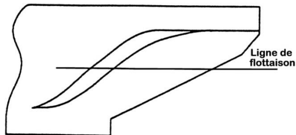
Figure 77 - Forme de l'avant non classique
