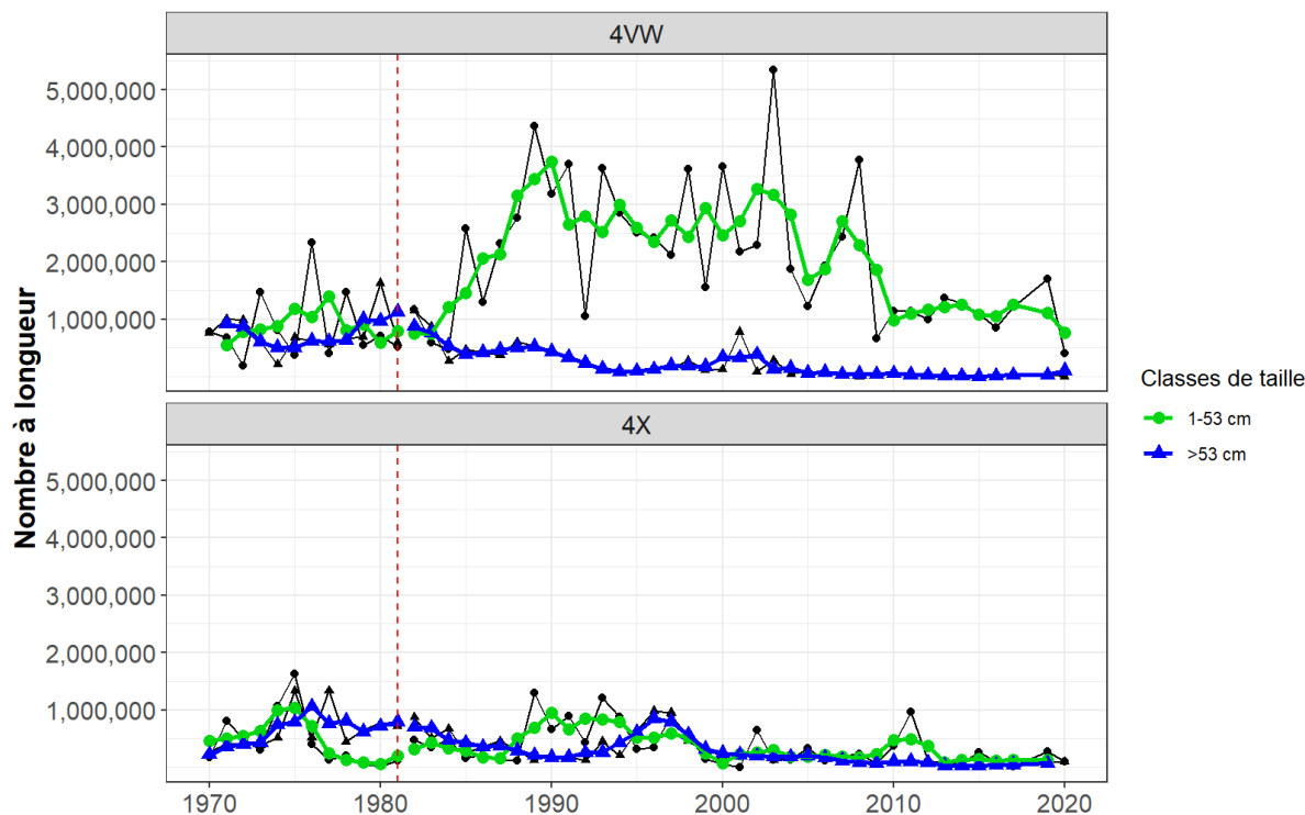
Figure 3. Abondance moyenne géométrique stratifiée sur trois ans des loups atlantiques immatures (1 à 53 cm) (triangles verts) et matures (> 53 cm) (cercles bleus) dans 4VW (graphique supérieur) et 4X (graphique inférieur) lors des relevés d'été des navires océanographiques du MPO (les discontinuités et la ligne pointillée indiquent un changement de navire et d'engin après 1981). Les lignes et symboles noirs représentent les valeurs annuelles.
