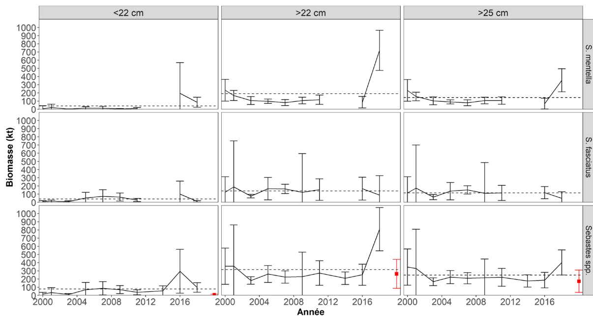
Figure 11. Biomasse chalutable en kilotonnes (kt, avec des intervalles de confiance à 95 %) de S. mentella , S. fasciatus et Sebastes spp. dans le relevé de l'unité 2 de 2000 à 2020, par classe de taille : 0-22 cm, >22 cm et > 25 cm. L'estimé de 2020 ne doit pas être interprété dans le contexte des séries chronologiques globales. Les lignes pointillées représentent la moyenne.
