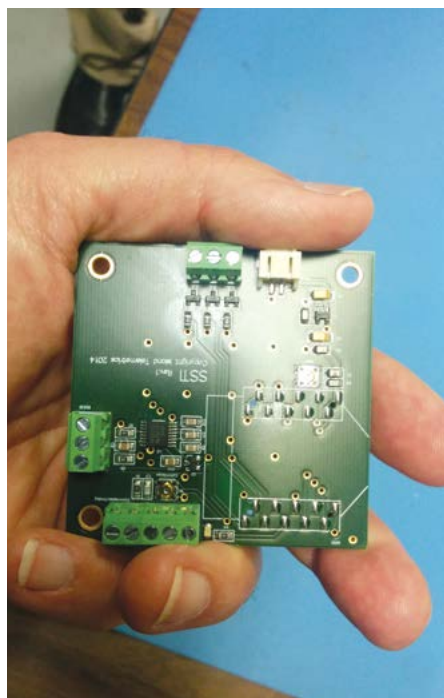
Carte mère personnalisée conçue pour commander le profileur muni d'un treuil, les divers capteurs de la qualité de l'eau et la télémétrie du système. Photo : Steve Morgan
