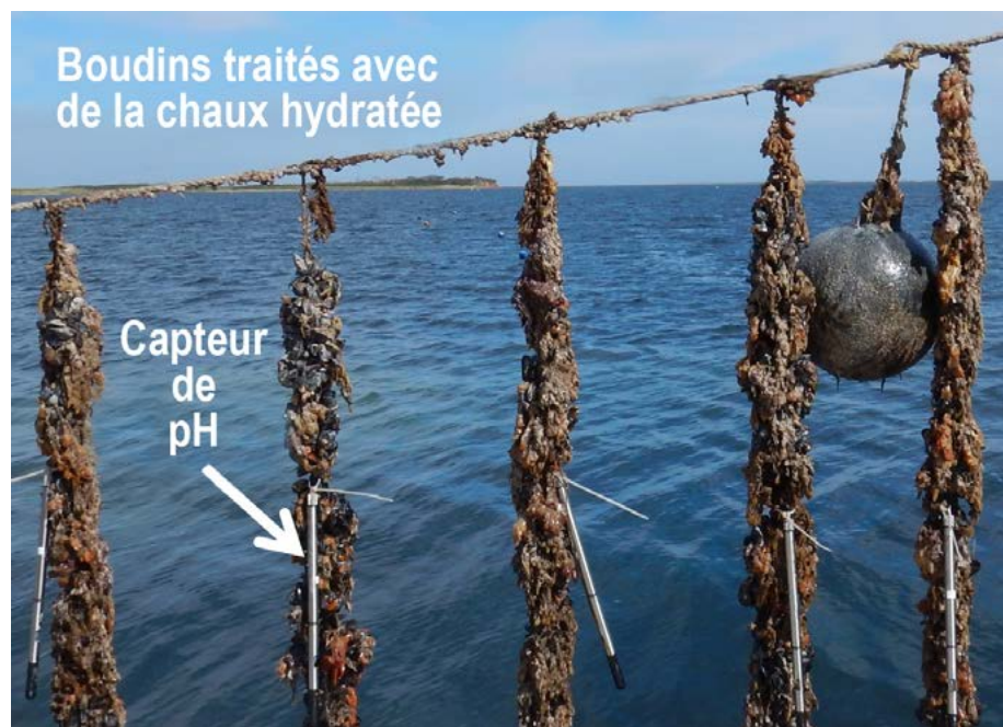
Boudins de moules dotés de capteurs de pH. Photo : Jonathan Hill
