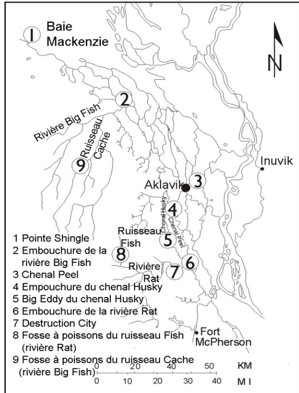
Figure 1. Emplacement des lieux de pêche, de surveillance, de frai et d'hivernage du Dolly Varden dans le réseau hydrographique de la rivière Rat dans le secteur du cours inférieur du fleuve Mackenzie (tiré de Harwood et al. 2009).
