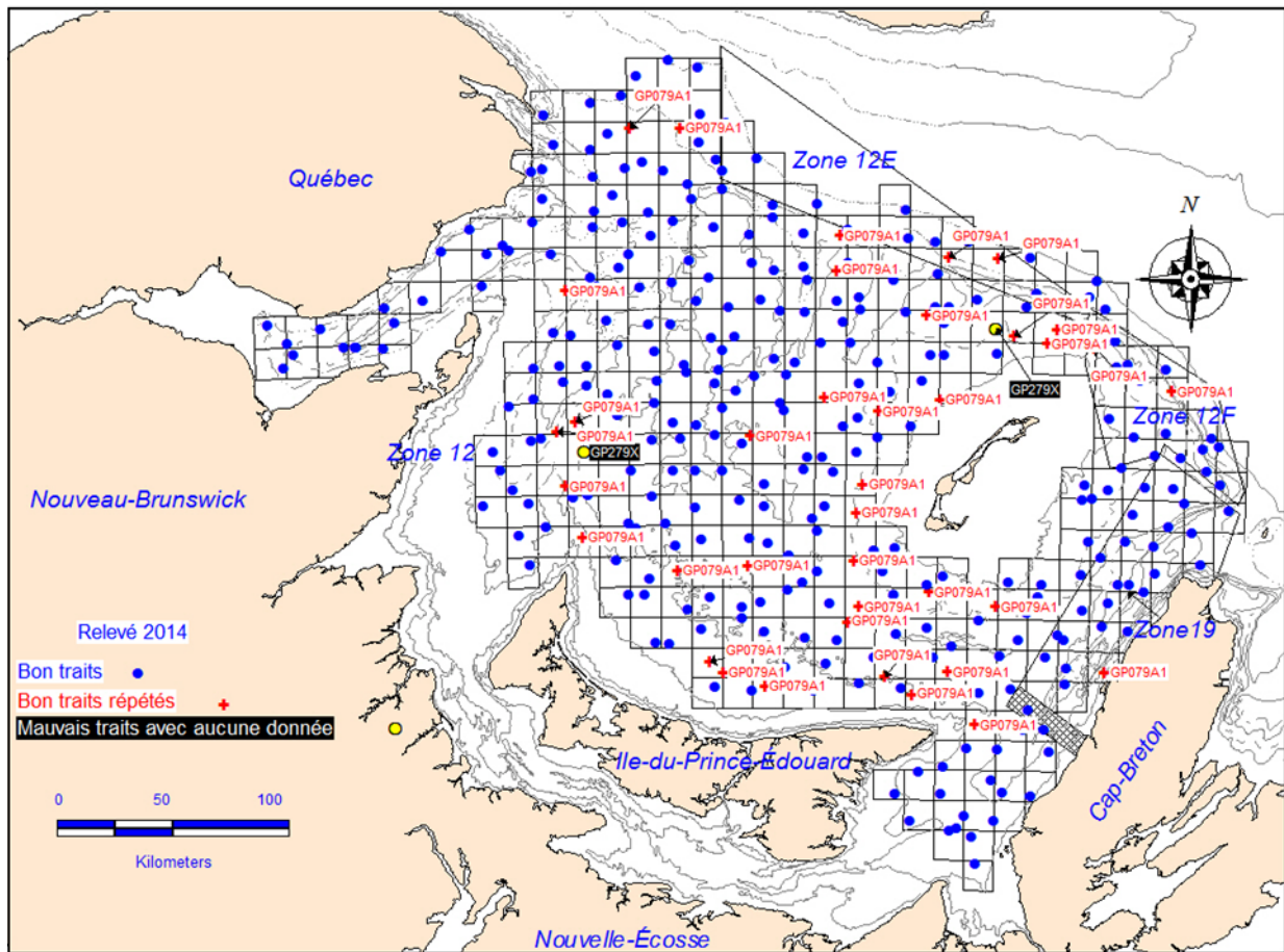
Figure 2. Positions des stations du relevé au chalut au crabe des neiges ( Chionoecetes opilio ) à l'intérieur du polygone d'estimation de 57 840 km 2 dans le sud du golfe du Saint-Laurent en 2014. Les points bleus sont des traits qui ont été réussis, les points rouges sont des traits qui ont été répétés et réussis et les points jaunes ( n = 2 ) sont des quadrilles qui ont été abandonnés.
