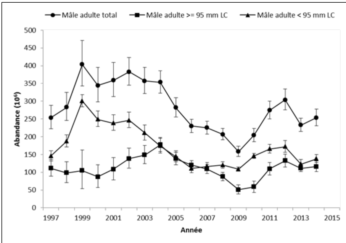
Figure 11. Abondance estimée des crabes des neiges ( Chionoecetes opilio ) mâles adultes dans le sud du golfe du Saint-Laurent, 1997 à 2014. LC = Largeur de carapace.
