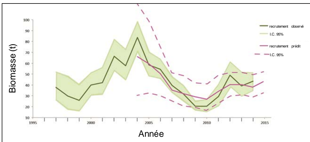
Figure 7. Comparaison entre le recrutement ( R-1 ) observé (moyenne avec intervalle de confiance de 95%) et prédit (moyenne avec intervalle de confiance de 95%) du crabe des neiges ( Chionoecetes opilio ) mâle selon le modèle Bayésien en se basant sur les pré-recrues (Surette et Wade 2006 ; Wade et al. 2013).
