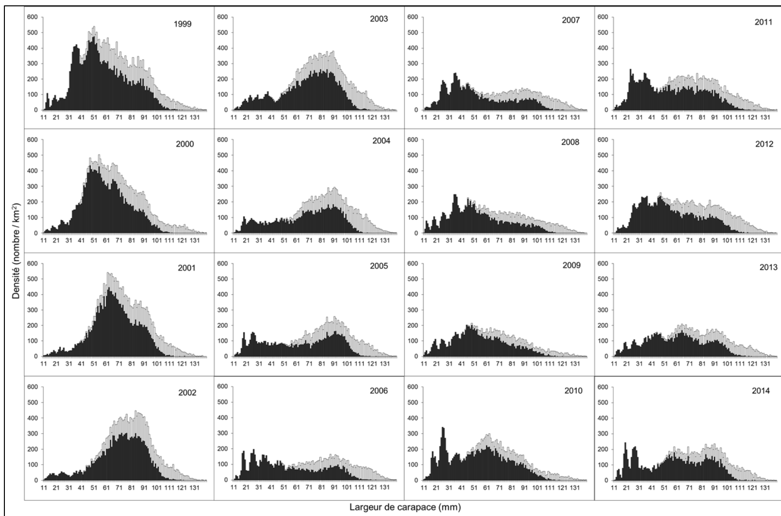
Figure 18. Distributions de fréquences de taille (par intervalle de 1 mm) des crabes des neiges ( Chionoecetes opilio ) mâles (barres blanches sont les mâles adultes et les barres noirs sont les mâles adolescents) basées sur les échantillons à partir des relevés au chalut effectués après la pêche dans le sud du golfe du Saint-Laurent, 1999 à 2014. Ces distributions représentent le nombre moyen de crabes mâles par km 2 basés directement sur les échantillons du relevé au chalut.
