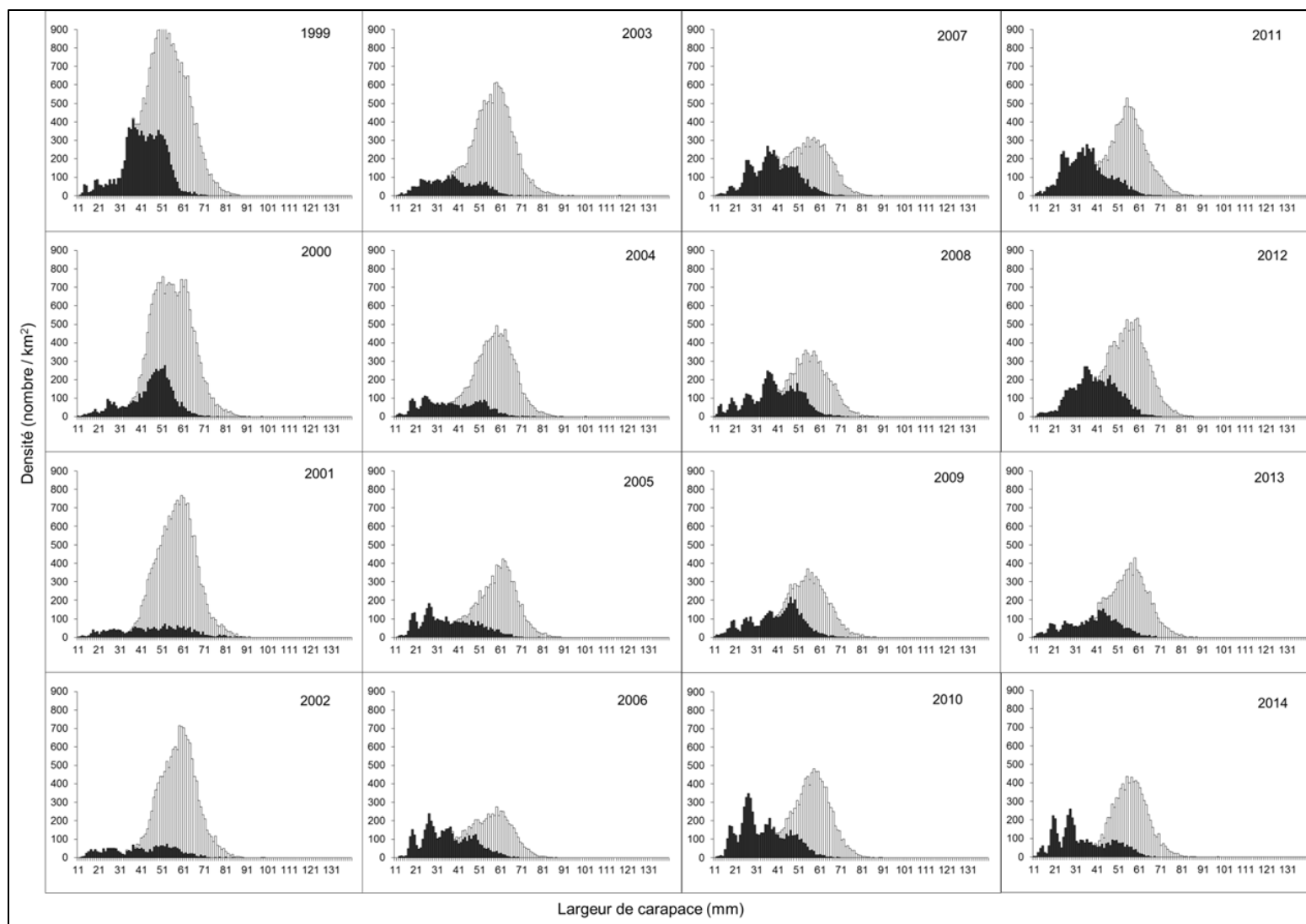
Figure 21. Distributions de fréquence des tailles (largeur de la carapace par intervalle de 1 mm) des femelles (barres blanches sont les femelles matures et les barres noirs sont les femelles pubescentes et immatures) de crabe des neiges ( Chionoecetes opilio ), basées sur les échantillons à partir des relevés au chalut effectués après la pêche dans le sud du golfe du Saint-Laurent, 1999 à 2014. Ces distributions représentent le nombre moyen de crabes femelles par km 2 basés directement sur les échantillons du relevé au chalut.
