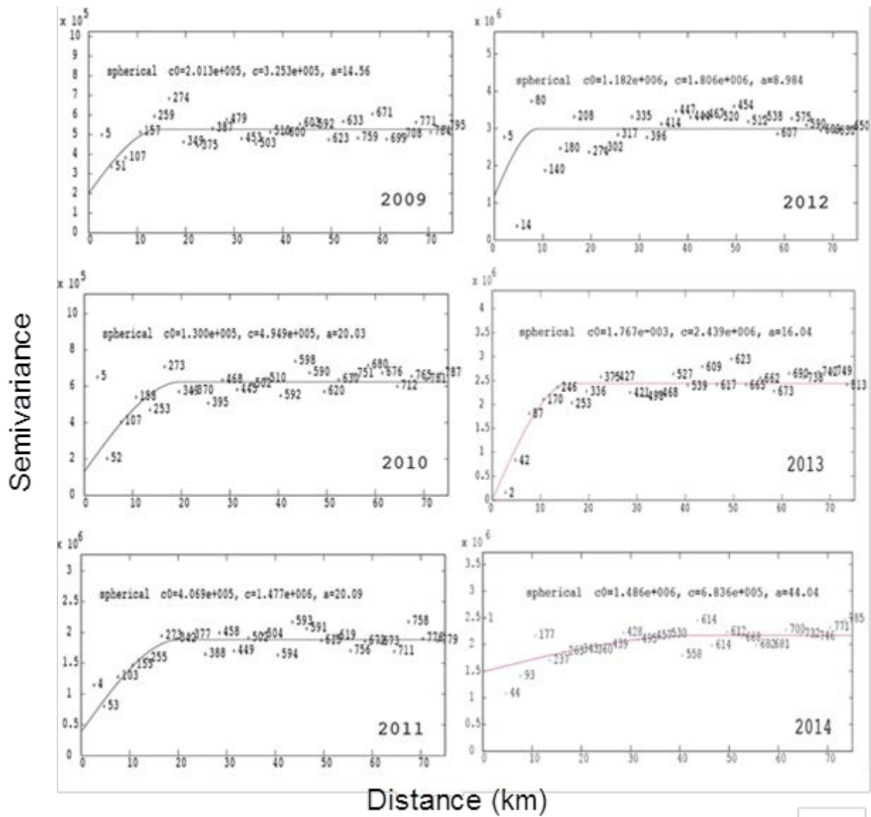
Figure 5. Modèles de variogrammes annuels pour les crabes des neiges ( Chionoecetes opilio ) mâles adultes de taille commerciale dans le sud du golfe du Saint-Laurent, 2009 à 2014. Indiqué est le nombre de paires d'observations utilisé dans le calcul de la semi-variance selon les distances décalées.
