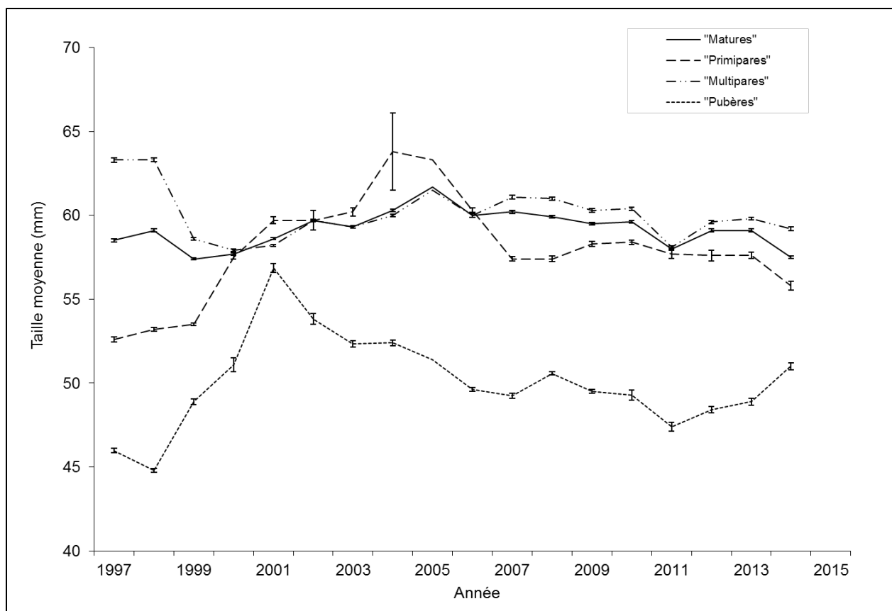
Figure 13. Taille moyenne (largeur de la carapace en mm) avec erreurs-types des femelles pubères, primipares, multipares et matures du crabe des neiges ( Chionoecetes opilio ) basée sur les échantillons provenant des relevés au chalut, 1997 à 2014.
