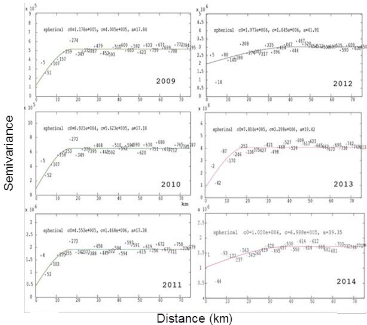
Figure 4. Modèles de variogrammes avec moyenne mobile sur trois ans pour les crabes des neiges ( Chionoecetes opilio ) mâles adultes de taille commerciale dans le sud du golfe du Saint-Laurent, 2009 à 2014. Indiqué est le nombre de paires d'observations utilisé dans le calcul de la semi-variance selon les distances décalées.
