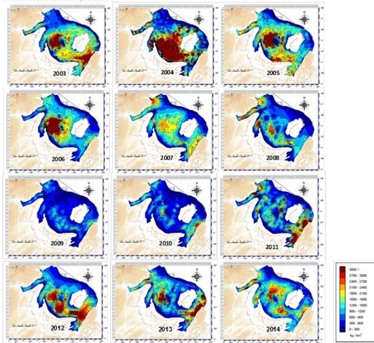
Figure 6. Contours de densités (kg par km 2 ) de crabes des neiges ( Chionoecetes opilio ) adultes mâles de taille commerciale ( \geq 95 mm de largeur de carapace) à partir des données des relevés au chalut effectués dans le sud du golfe du Saint-Laurent, 2003 à 2014.
