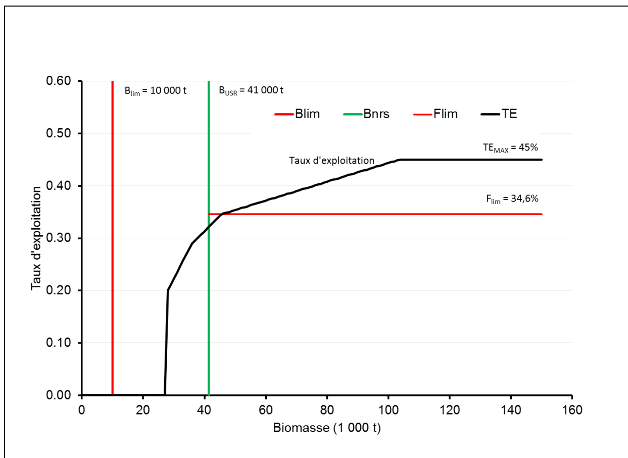
Figure 16. Règle de décision proportionnelle (variante 4) conforme à l'approche de précaution pour la pêche au crabe des neiges ( Chionoecetes opilio ) dans le sud du golfe du Saint-Laurent. B_{lim} = Le niveau de référence limite pour la biomasse ; F_{lim} = Le niveau de référence limite pour le taux d'exploitation ; B_{NRS} = Le point de niveau de référence supérieur du stock. TE = Les taux d'exploitations basés sur la règle de décision proportionnelle (variante 4) (MPO 2014b).
