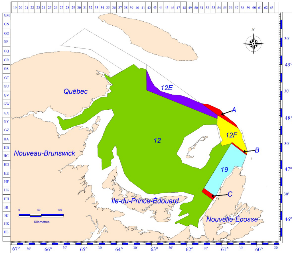
Figure 3. Le polygone d'estimation de 57 840 km 2 utilisé pour l'évaluation de stock de crabe des neiges ( Chionoecetes opilio ) en 2014 dans le sud du golfe du Saint-Laurent (toutes les régions colorées) et les polygones d'estimation correspondants pour les quatre zones de pêche (12, 12E, 12F et 19). La zone non-assignée au nord des zones 12E et 12F (étiquetée A) et les zones tampons (étiquetées B et C) sont aussi indiquées.
