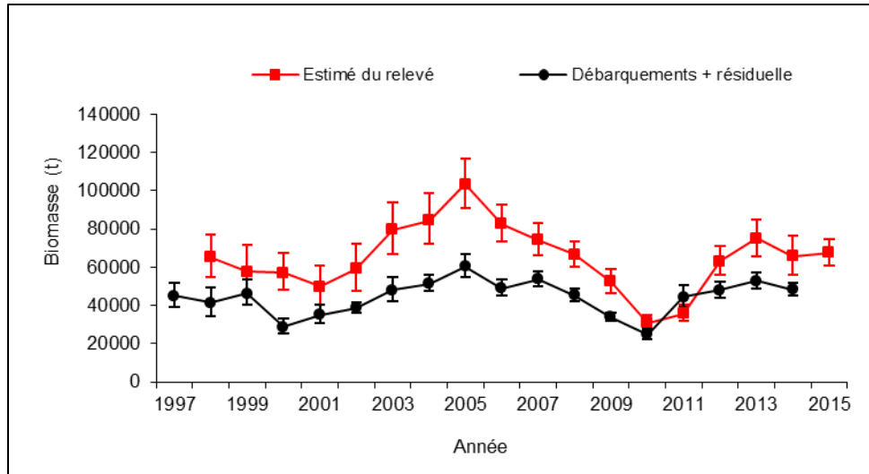
Figure 10. Comparaison de la biomasse calculée après la pêche (somme de la biomasse résiduelle et les débarquements à l'année t+1 ) et la biomasse avant la pêche des crabes des neiges ( Chionoecetes opilio ) mâles adultes de taille commerciale (la somme du recrutement et la biomasse résiduelle à l'année t ) estimées par le relevé au chalut dans le sud du golfe du Saint-Laurent.
