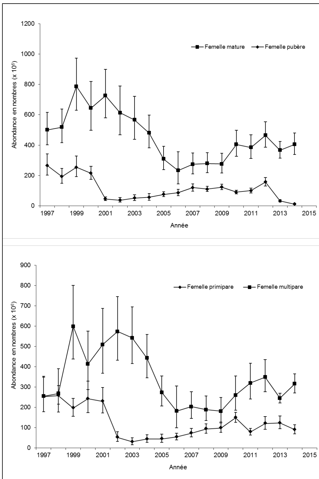
Figure 12. Abondance des femelles pubères, primipares, multipares et matures du crabe des neiges ( Chionoecetes opilio ) dans le sud du golfe du Saint-Laurent, 1997 à 2014.
