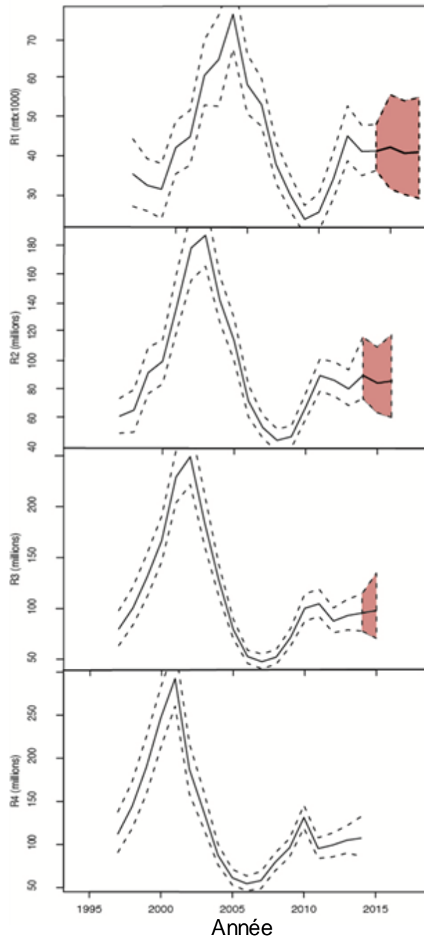
Figure 15. Abondances (moyenne avec intervalles de confiance à 95%), de recrutement ( R ) de crabe des neiges, ( Chionoecetes opilio ), pour R(j) , où j = 1, \dots, 4 années avant le recrutement à la pêche. Les parties ombragées représentent les projections d'abondance à partir du modèle Bayésien (Wade et al. 2014).
