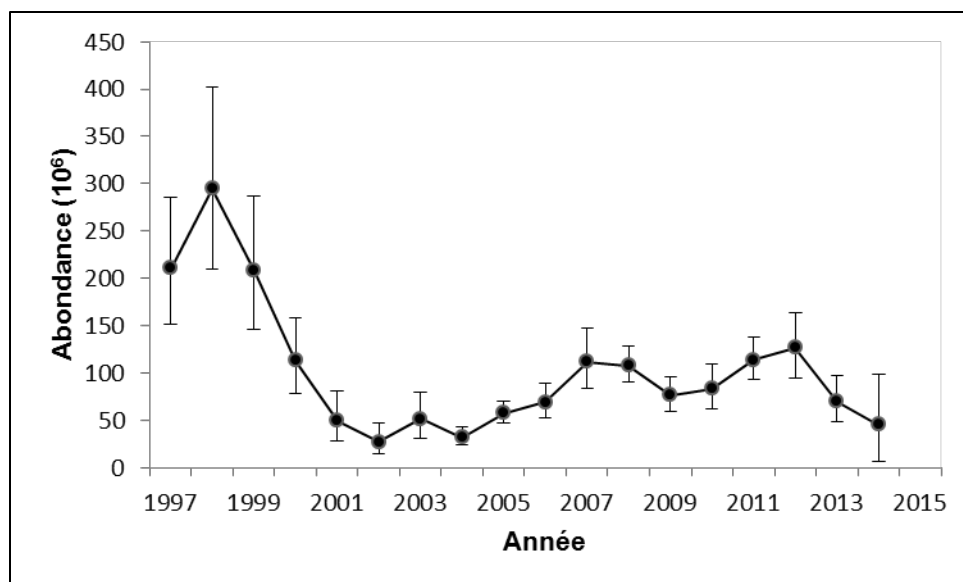
Figure 19. Indices d'abondance des petits crabe des neiges ( Chionoecetes opilio ) mâles adolescents avec largeur de carapace de 34 à 44 mm estimées à partir des données des relevés au chalut dans le sud du golfe du Saint-Laurent, 1997 à 2014. Ces crabs vont atteindre la taille commerciale dans environ six ans.
