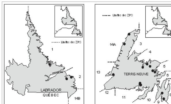
Figure 1. Emplacements évalués dans la Région de Terre-Neuve-et-Labrador
