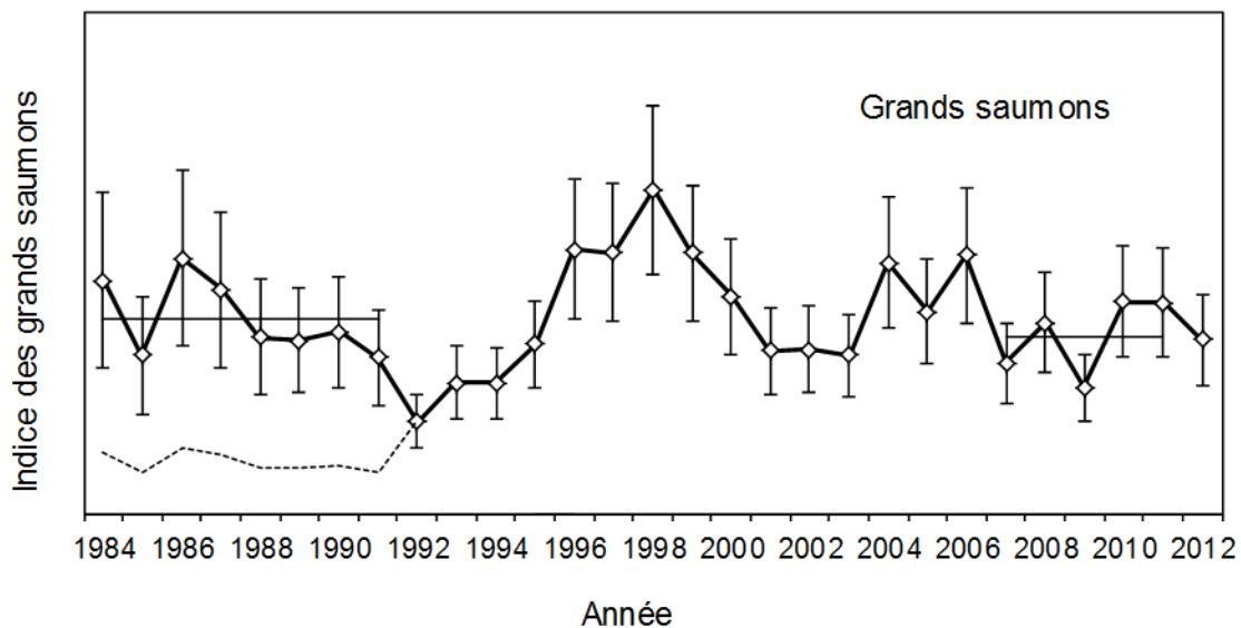
Figure 7. Tendances relatives à l'abondance des grands saumons de l'Atlantique à Terre-Neuve, 1984 à 2012. Les montaisons de saumons de 1984 à 1991 ont été corrigées afin de tenir compte de l'exploitation en mer. Les lignes horizontales illustrent l'indice de l'abondance moyen pour les périodes allant de 1984 à 1991 et de 2007 à 2011. Les lignes verticales représentent \pm un écart type de \pm 1 . Les lignes en pointillé fin représentent les montaisons dont l'exploitation n'a pas été ajustée pour la période allant de 1984 à 1991.
