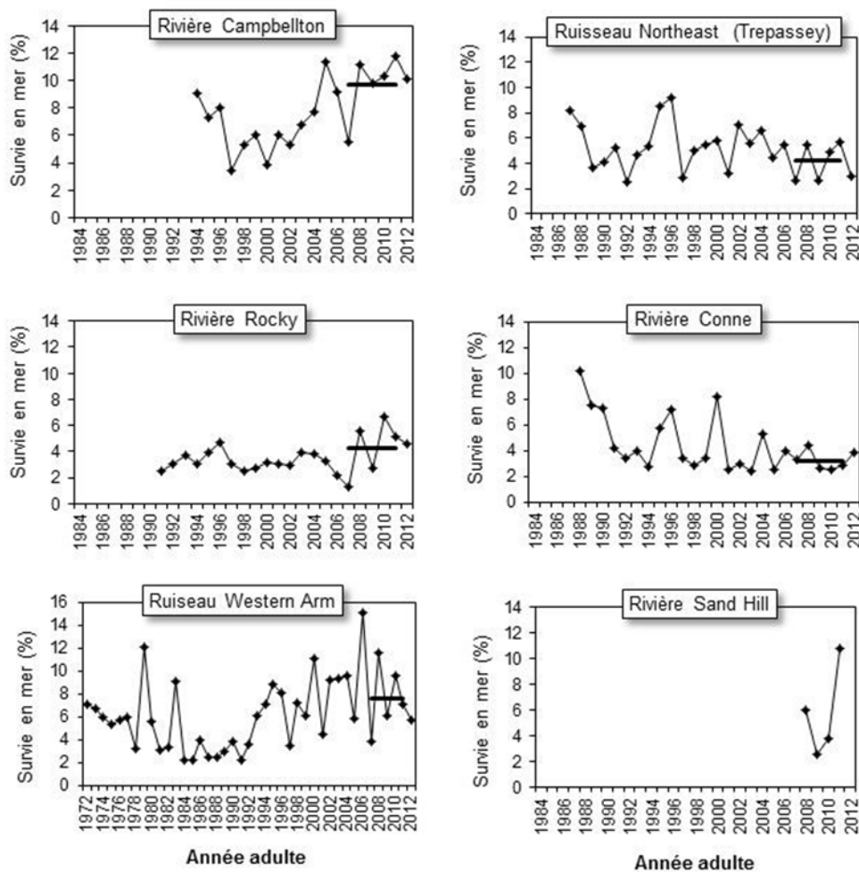
Figure 9. Taux de survie en mer du stade de saumoneau jusqu'au stade de montaison du petit saumon adulte dans plusieurs rivières de Terre-Neuve-et-Labrador. Ces taux de survie n'ont pas été ajustés pour tenir compte de l'exploitation en mer pendant la pêche commerciale du saumon (avant 1992) ou de la pêche autochtone au Labrador. Par conséquent, les valeurs représentent la survie du saumon lorsqu'il retourne dans la rivière. Les lignes horizontales pleines représentent la moyenne des cinq années précédentes (2007-2011).
