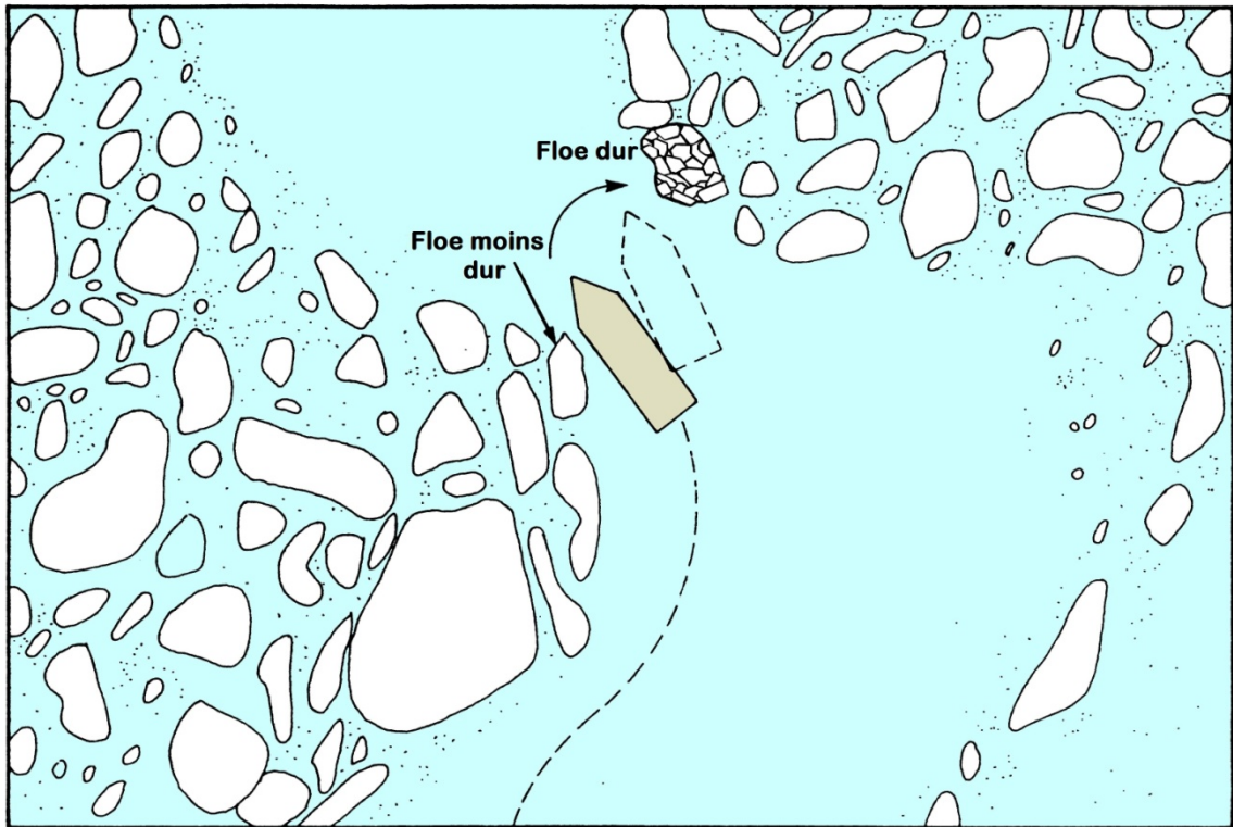
Figure 50 : Danger d'une manœuvre de virage dans un chenal en zone de glaces
