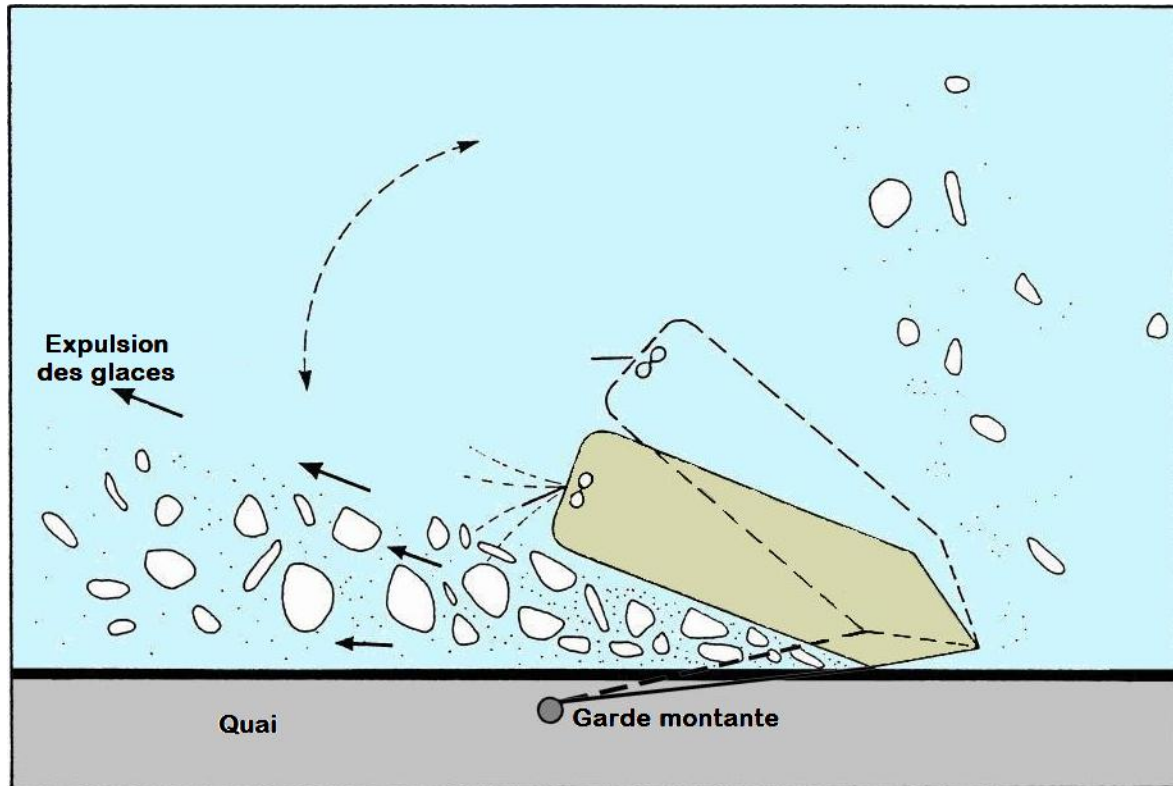
Figure 54 Accostage : expulsion des glaces par le remous pendant que la proue est amarrée avec une garde montante
