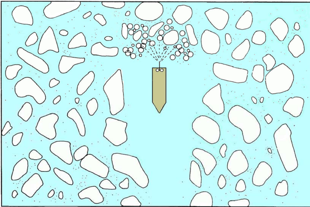
Figure 51: Manœuvre de recul dans les glaces : barre à zéro, marche arrière très lente
