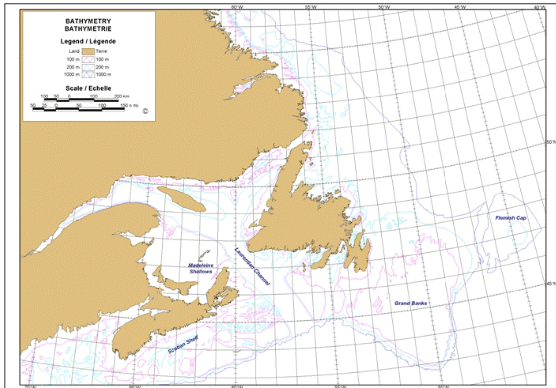
Figure 31 : Bathymétrie de la Côte est (Carte courtoisie d'Environnement Canada)
