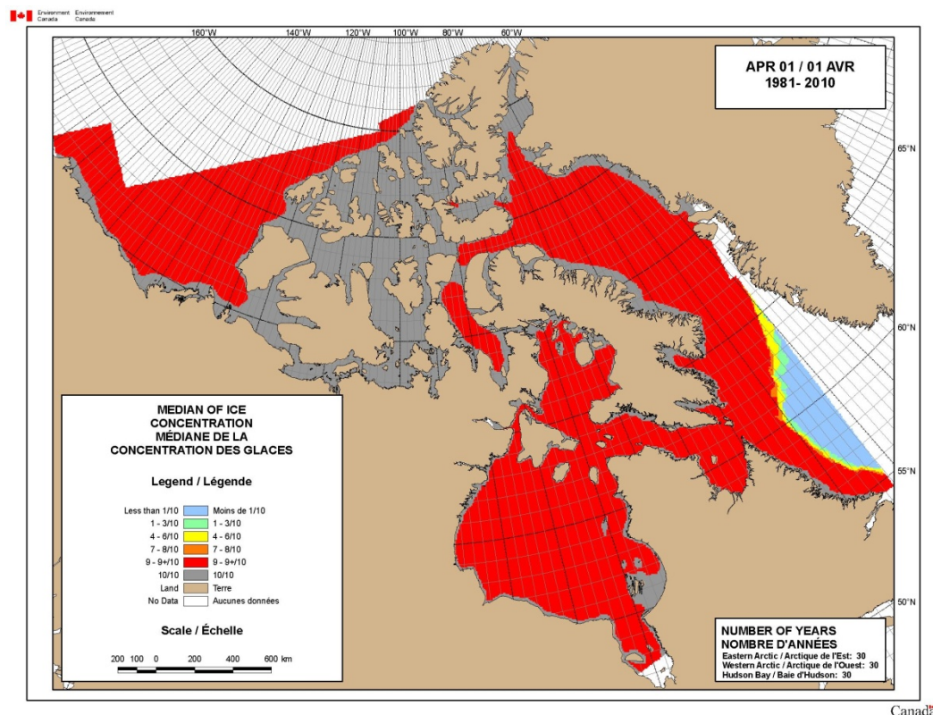
Figure 41 : Concentration médiane de glace dans l'Arctique canadien
