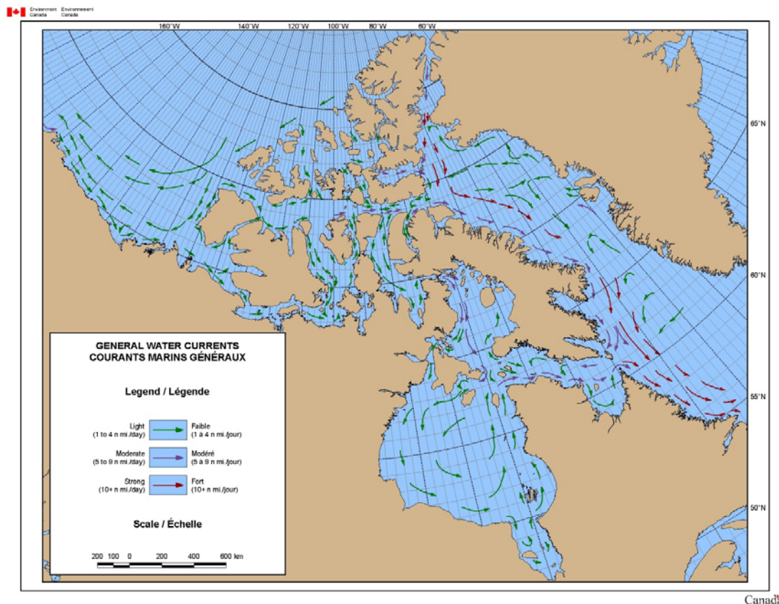
Figure 36 : Courants marins généraux dans les eaux du Nord
