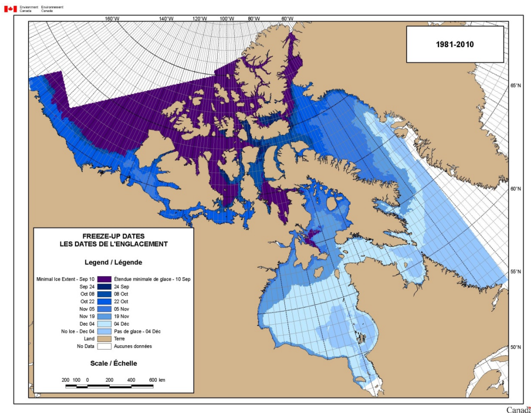
Figure 39 Dates de l'englacement dans l'Arctique canadien
