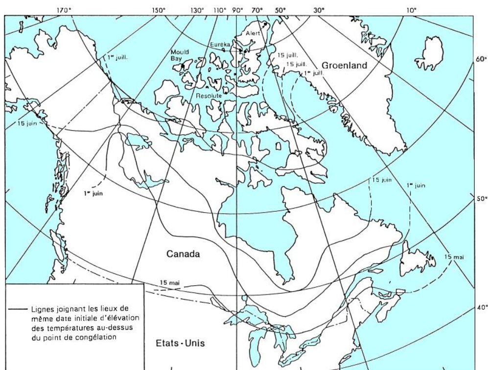
Figure 15 : Dates auxquelles les températures journalières moyennes s'élèvent au-dessus de 0 °C
