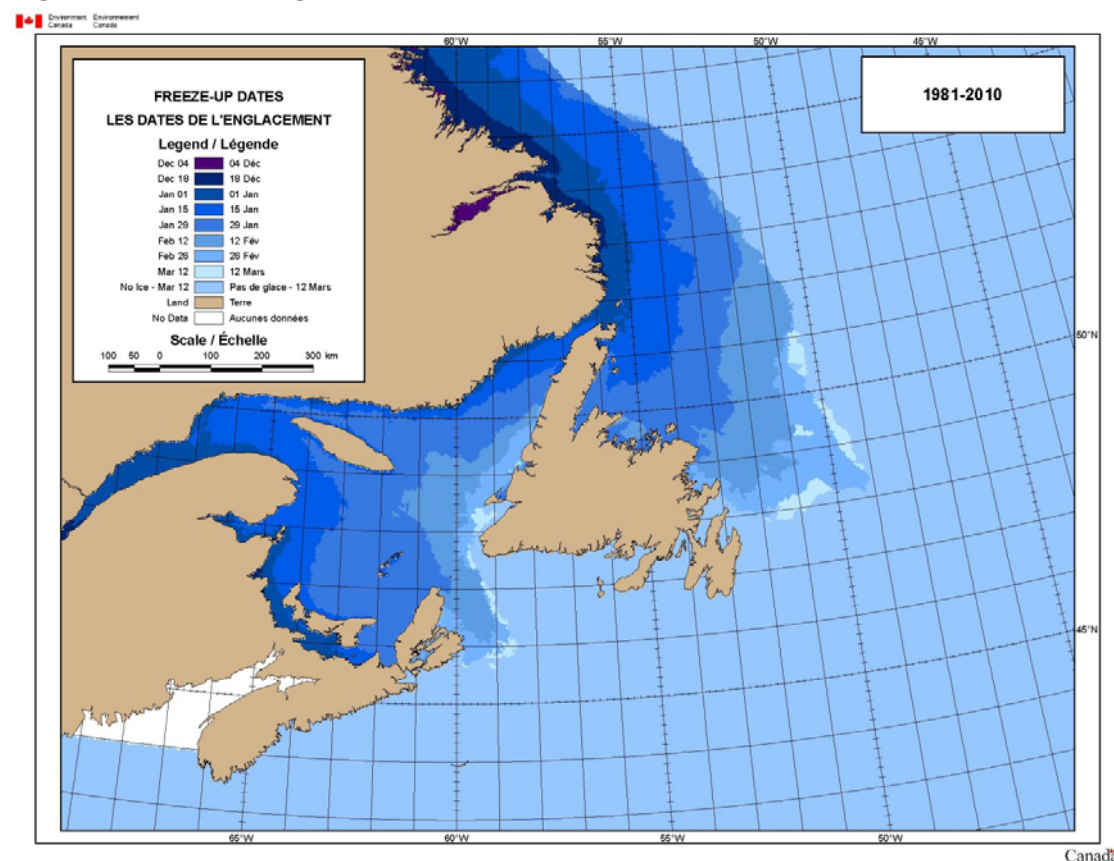
Figure 34 : Dates d'englacement
