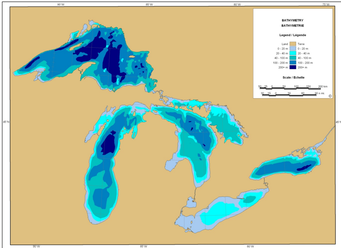
Figure 25 : Bathymétrie des Grands Lacs (Carte courtoisie d'Environnement Canada)
