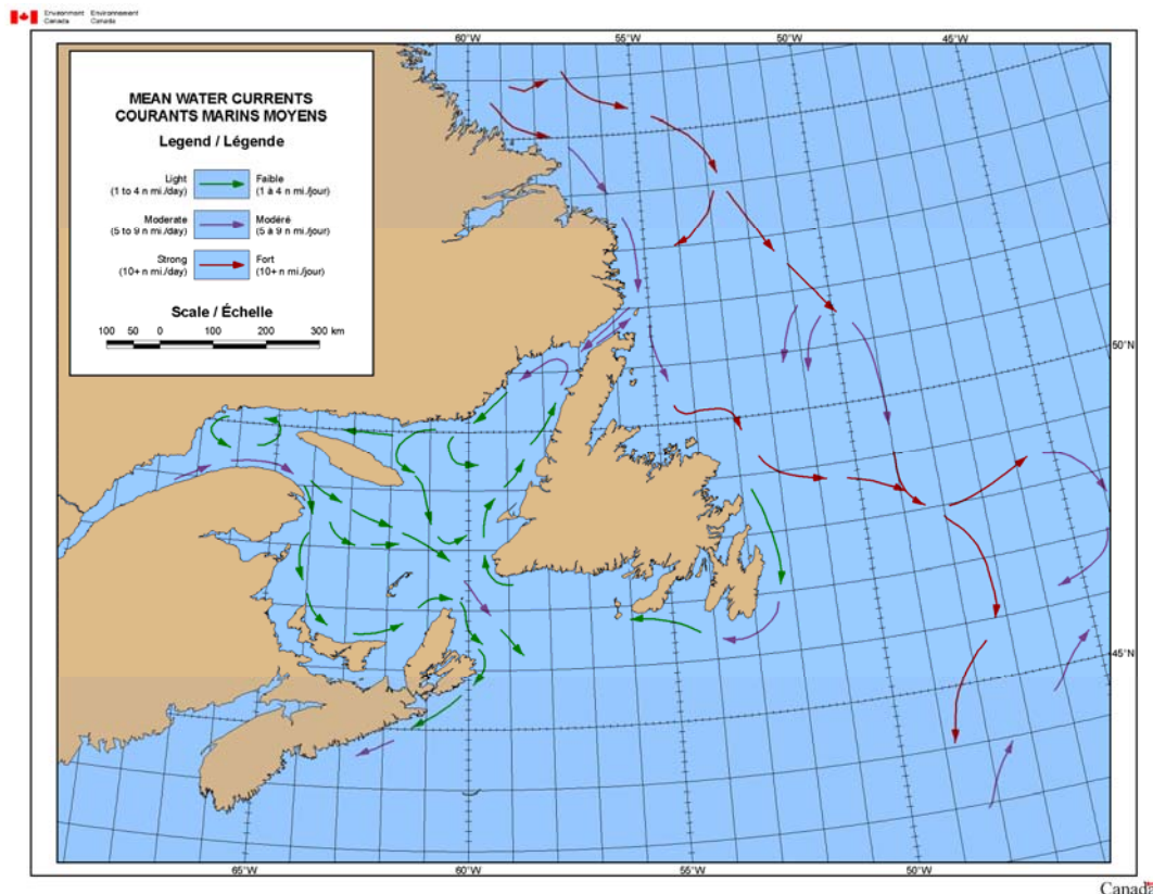
Figure 30 : Courants de surface sur la côte Est canadienne
