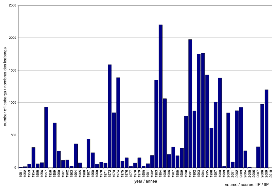
Figure 24 Nombre annuel d'icebergs franchissant le 48° de latitude Nord
