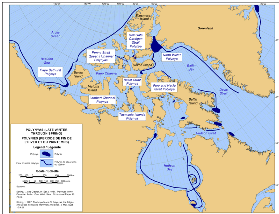
Figure 37 : Disposition des polynies récurrentes de l'Arctique canadien
