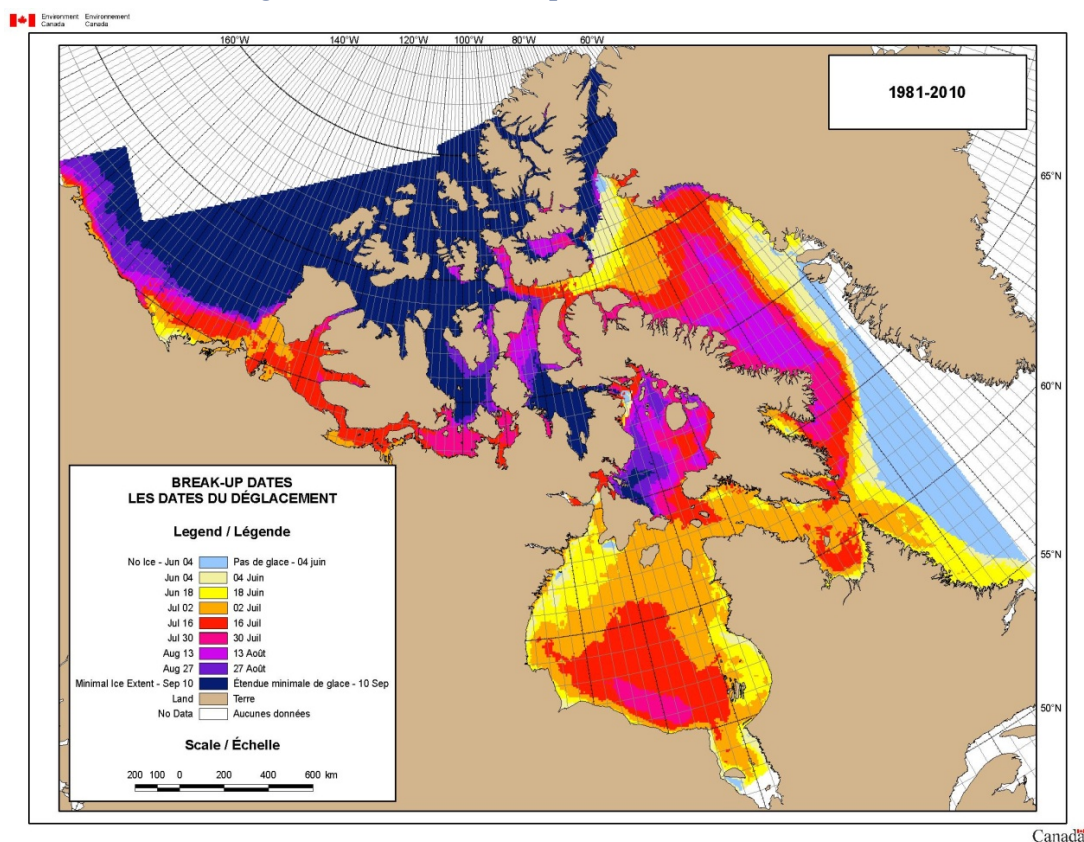
Figure 38 : Dates du déglacement dans l'Arctique canadien
