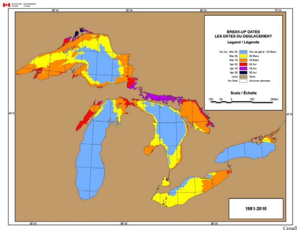
Figure 27 : Dates du déglacement pour les Grands Lacs
