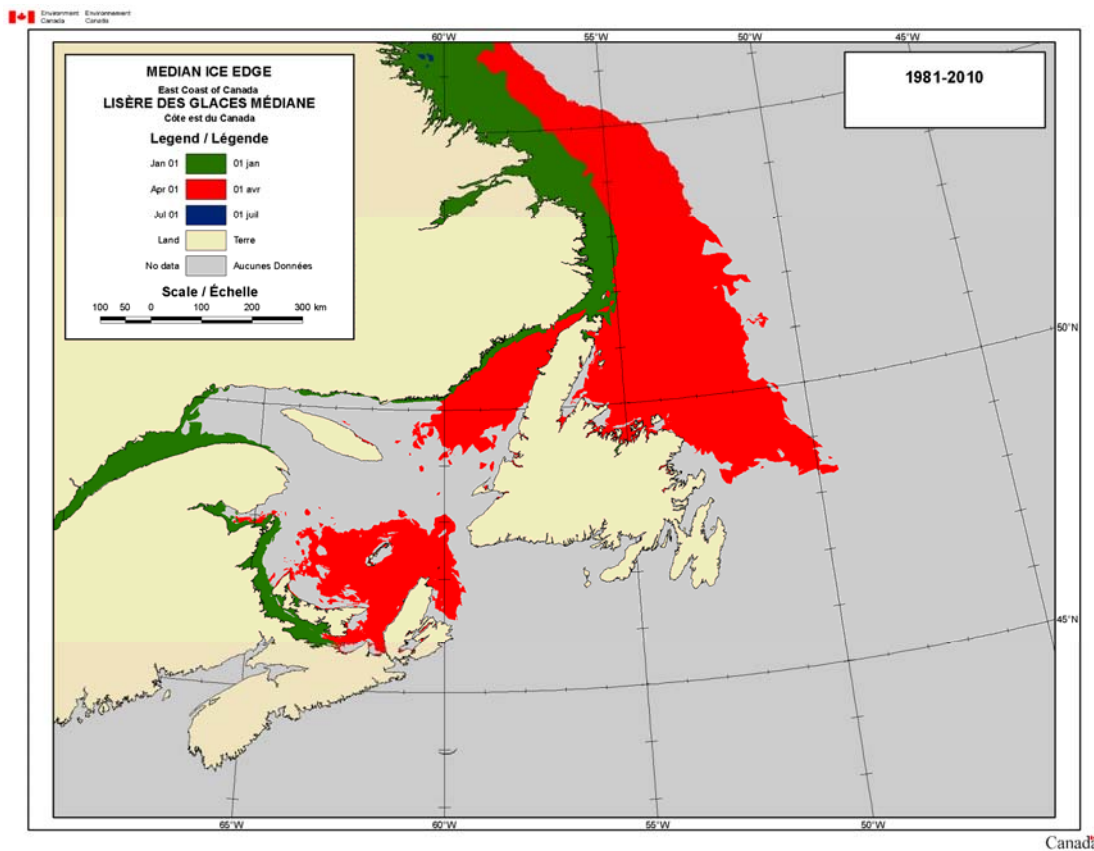
Figure 32 : Position de la lisière des glaces en janvier, avril et juillet sur la côte Est du Canada
