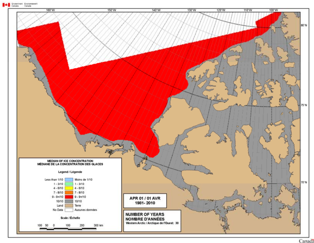
Figure 42 : Étendue des glaces de mer au milieu de l'hiver dans la mer de Beaufort
