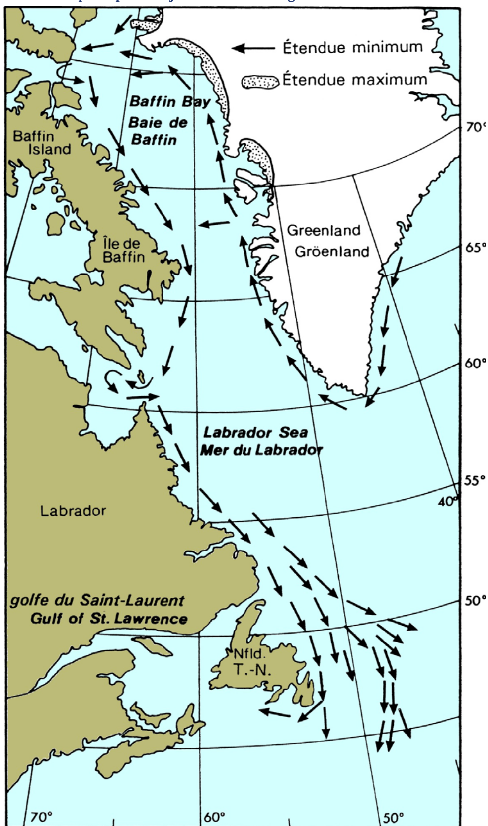
Figure 22 Sources et principales trajectoires des icebergs dans les eaux canadiennes
