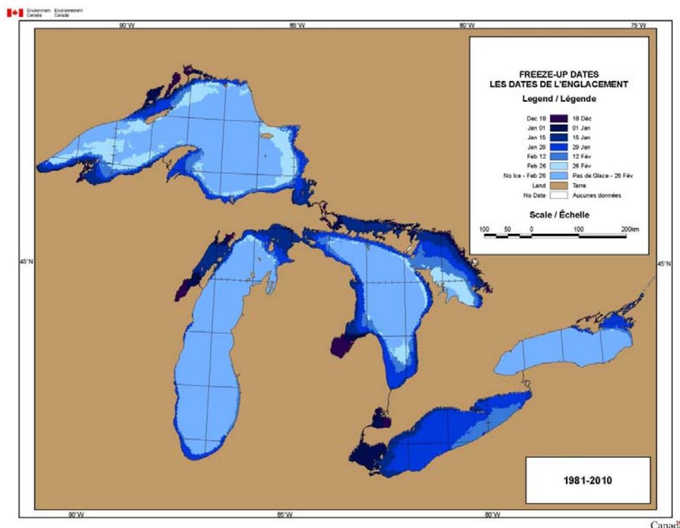
Figure 26 Dates d'englacement pour les Grands Lacs
