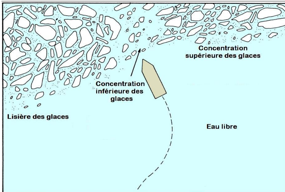
Figure 49 : Procédure adéquate pour aborder un champ de glace : approche lente et perpendiculaire à la lisière
