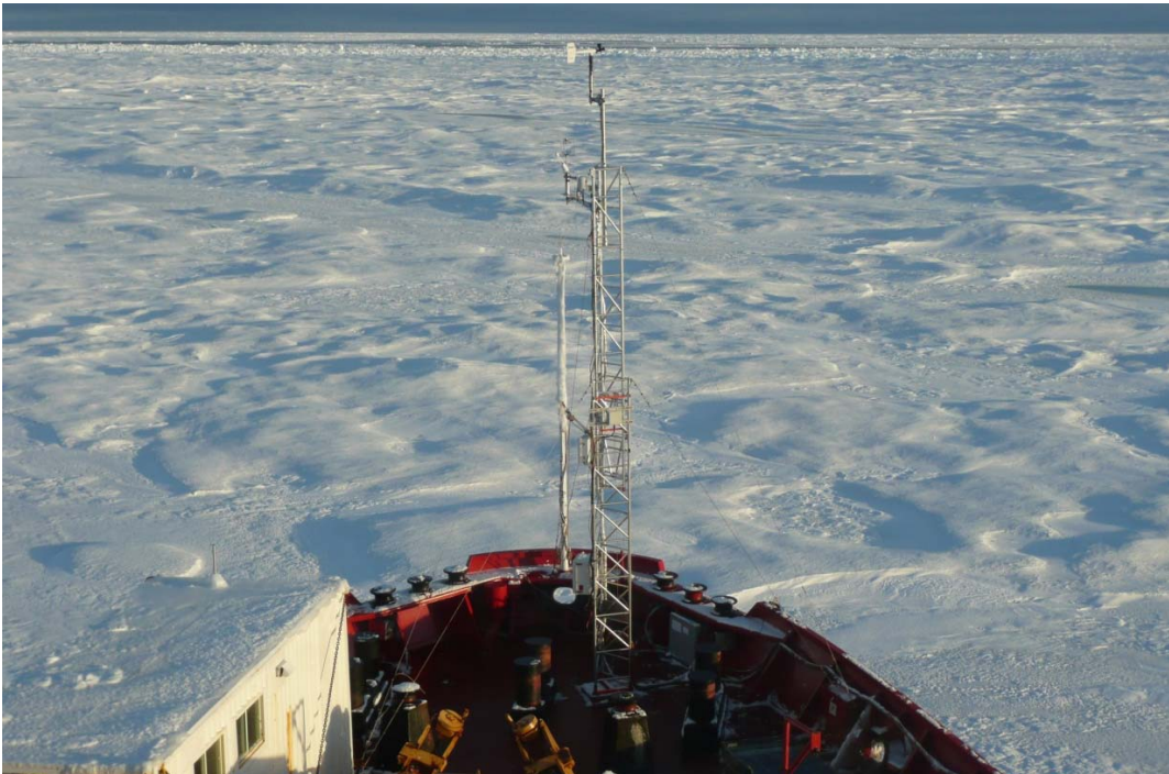
Figure 72 : Exemple de glace de deuxième année
