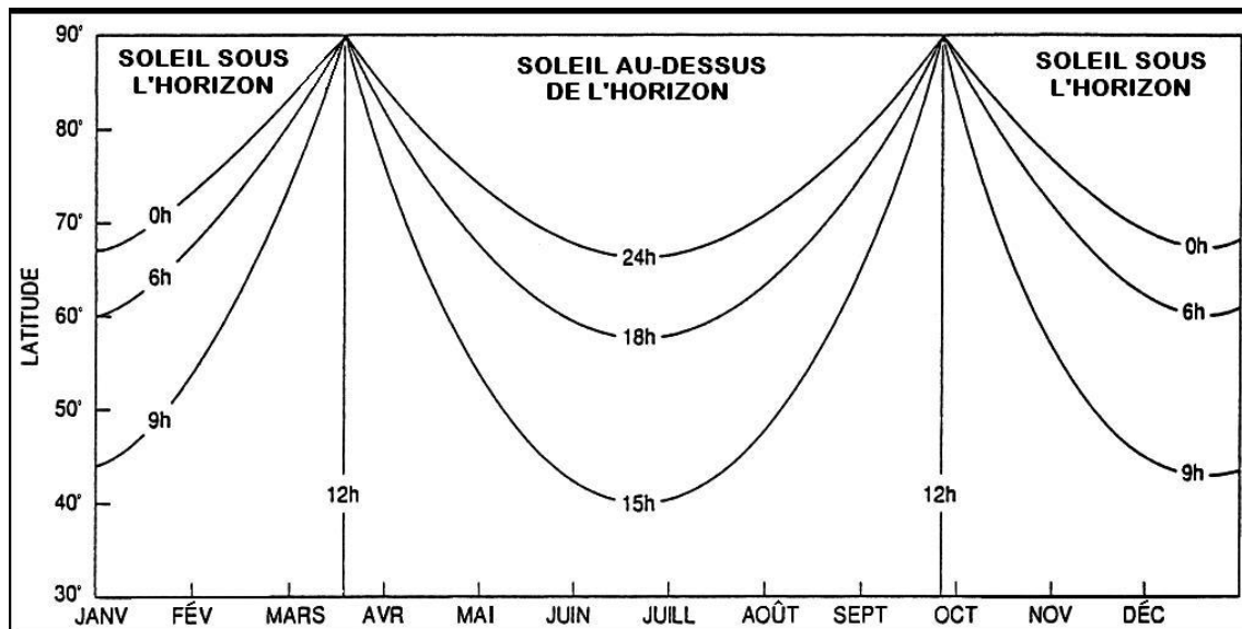
Figure 18 : Variabilité saisonnière du jour selon la latitude et le mois
