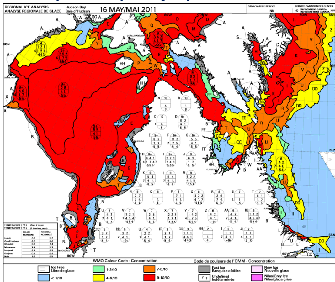
Figure 40 : Exemple de carte composite des glaces pour la baie et le détroit d'Hudson
