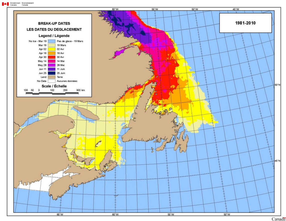
Figure 35 : Dates de déglacement
