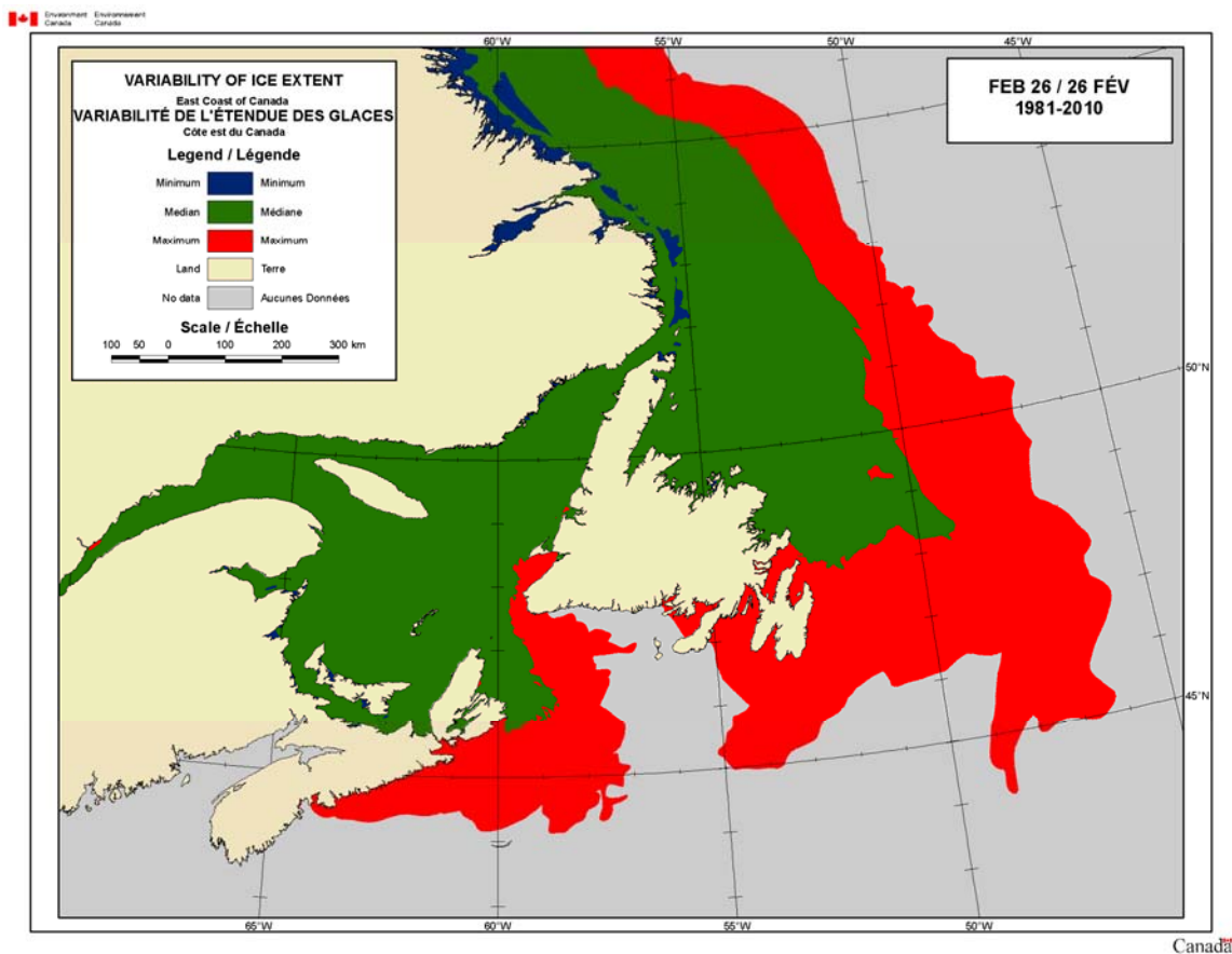
Figure 33 : Variabilité de l'étendue des glaces sur la côte Est
