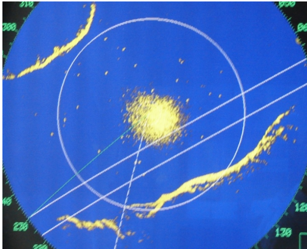
Figure 57 : Image produite au moyen d'un radar en bande X courant
