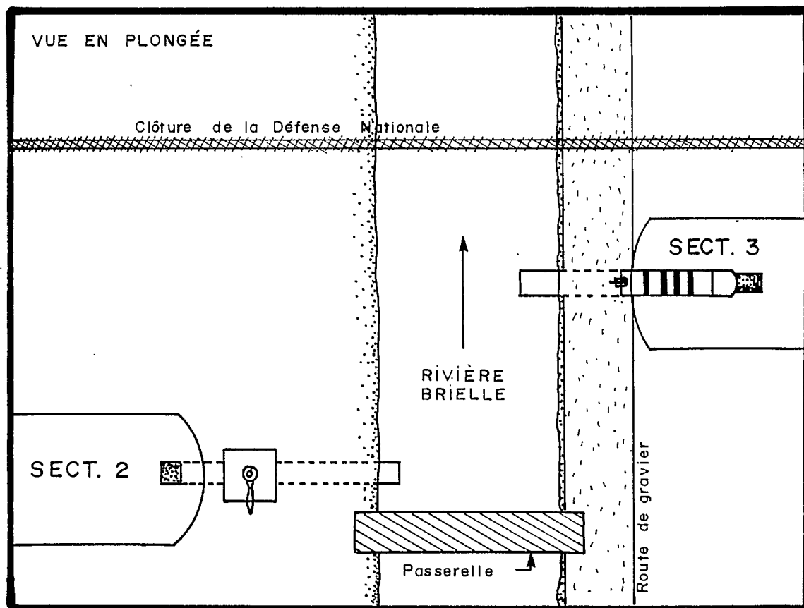
Figure 4: Présentation schématique et localisation des pompes.
