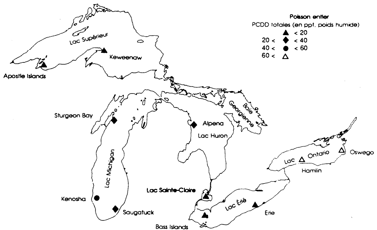
Distribution spatiale des polychloro-dibenzo-p-dioxines totales chez le poisson entier des Grands Lacs
