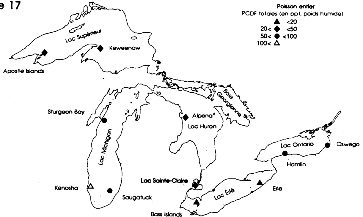
Distribution spatiale des polychloro-dibenzofuranes totaux chez le poisson entier des Grands Lacs
