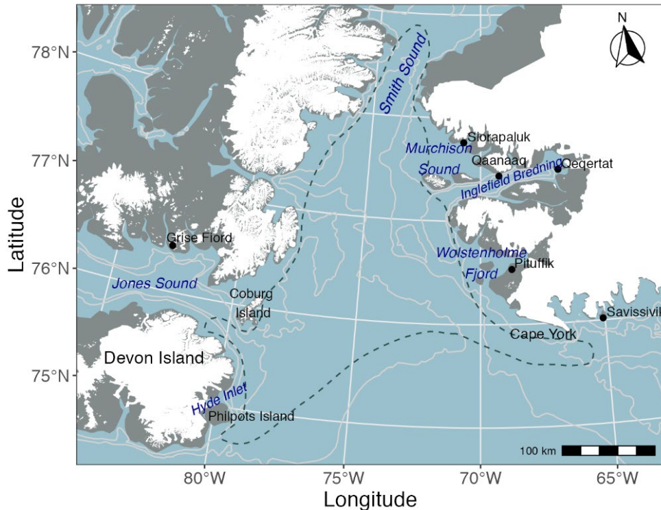
Assiliaq 2. Pikialasorsuaq qanillillugu, immap naqqata ilusaa itissutsinut 200-500 meterinut killingi ilanngullugit (aallerfik: Natural Resources Canada), matumanilu nalunaarusiami kangerluit, qeqertat imartallu pingaarutillit taaneqartut.
