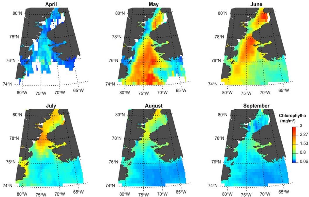
Assiliaq 4. Pikialasorsuarmi fytoplanktonit ukiup ingerlanerani naaruttortarnerisa allanngorartarneri, Uuttuusersuilluni ungasianiit klorofyl a kimittussusaata malinnaaffiginera tunngavigalugu. Qalipaait takutippaat, klorofyli a kimittussusaat assigiinngitsut (aappalaartoq = kimittunerpaq maajimi sumiiffiup qiterpasissuani naaruttornernik takutitsisoq). Immap assingisa pinngoraqqaarnerup annertussusivia annikinaarlugu takutikkunarpaat, takutiinnarpaami immap qaani klorofyli a immap iluani sikullu ataani pinngorartitseqqaarneq takutinnagu. Ikerinnarmi klorofyli a pillugu ilisimasat suli killeqarput (Aallerfik: Marchese et al. 2017).
