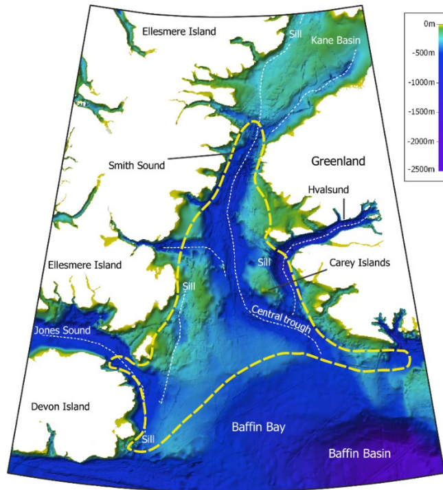
Assiliaq 3. Pikialasorsuarmi eqqaanilu immap naqqata ilusaa (meterinngorlugu). Qoororsuit itisuut kipisaartunik qaqortunik titartorsimapput qooqqullu sanimukaartut (sills) nalunaarsimallutik (aallerfik International Bathymetric Chart of the Arctic Ocean (IBCAO) ver. 4 ).
